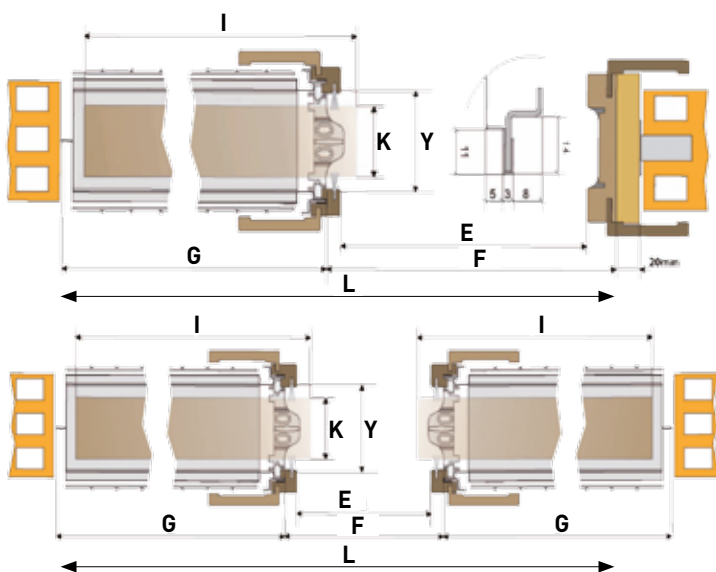
Sezione orizzontale Anta Singola
